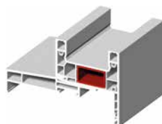
Appui rapporté de 135 mm total en 2 rails (réf. T1410)
